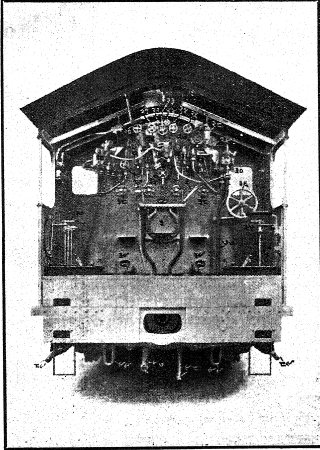
चित्र १७२-डाइवर के काम के सब यंत्र सामने लगे हैं।
